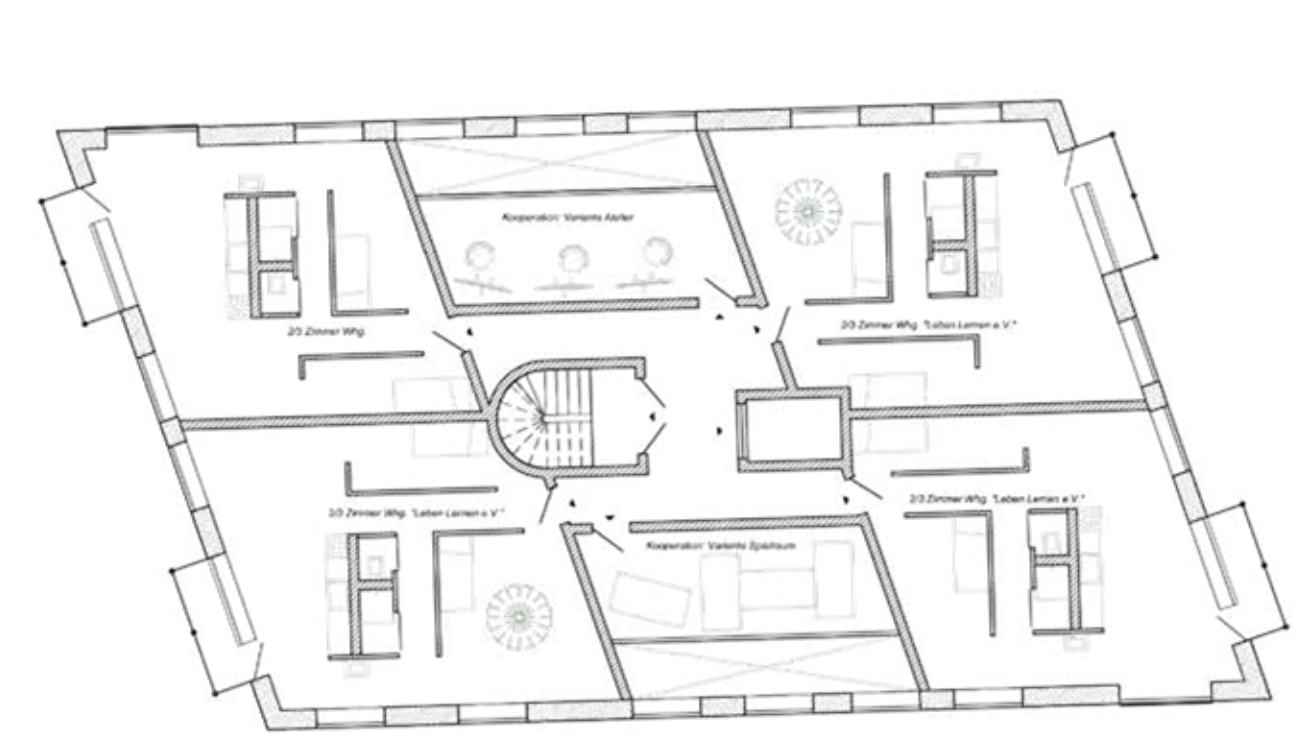
Grundriss 3. Obergeschoss M 1:200
