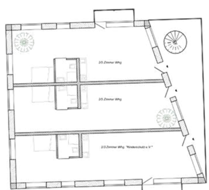
Grundriss 1. Obergeschoss M 1:200
