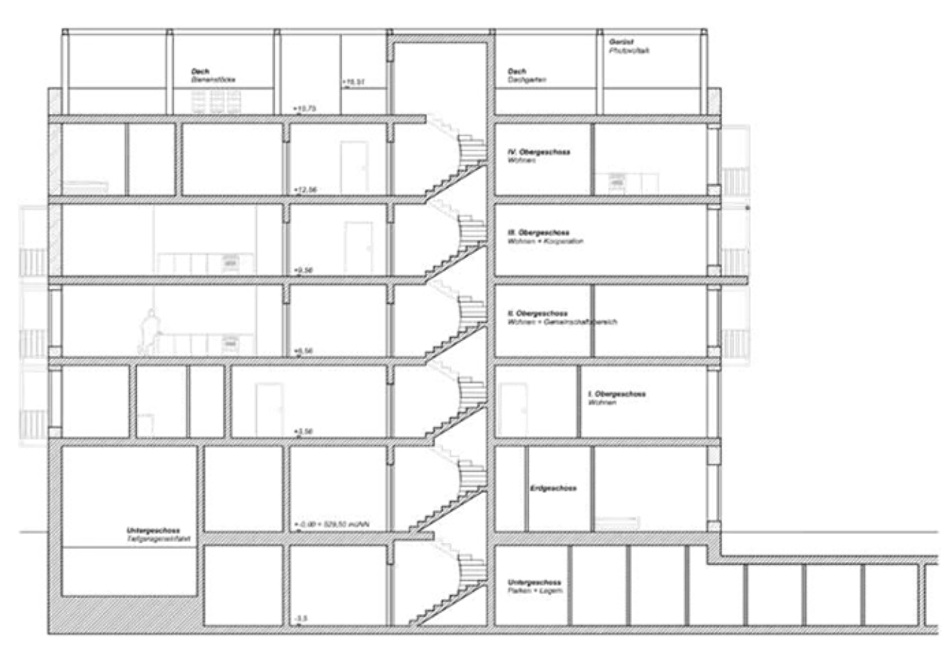
Schnitt B-B M 1:200
