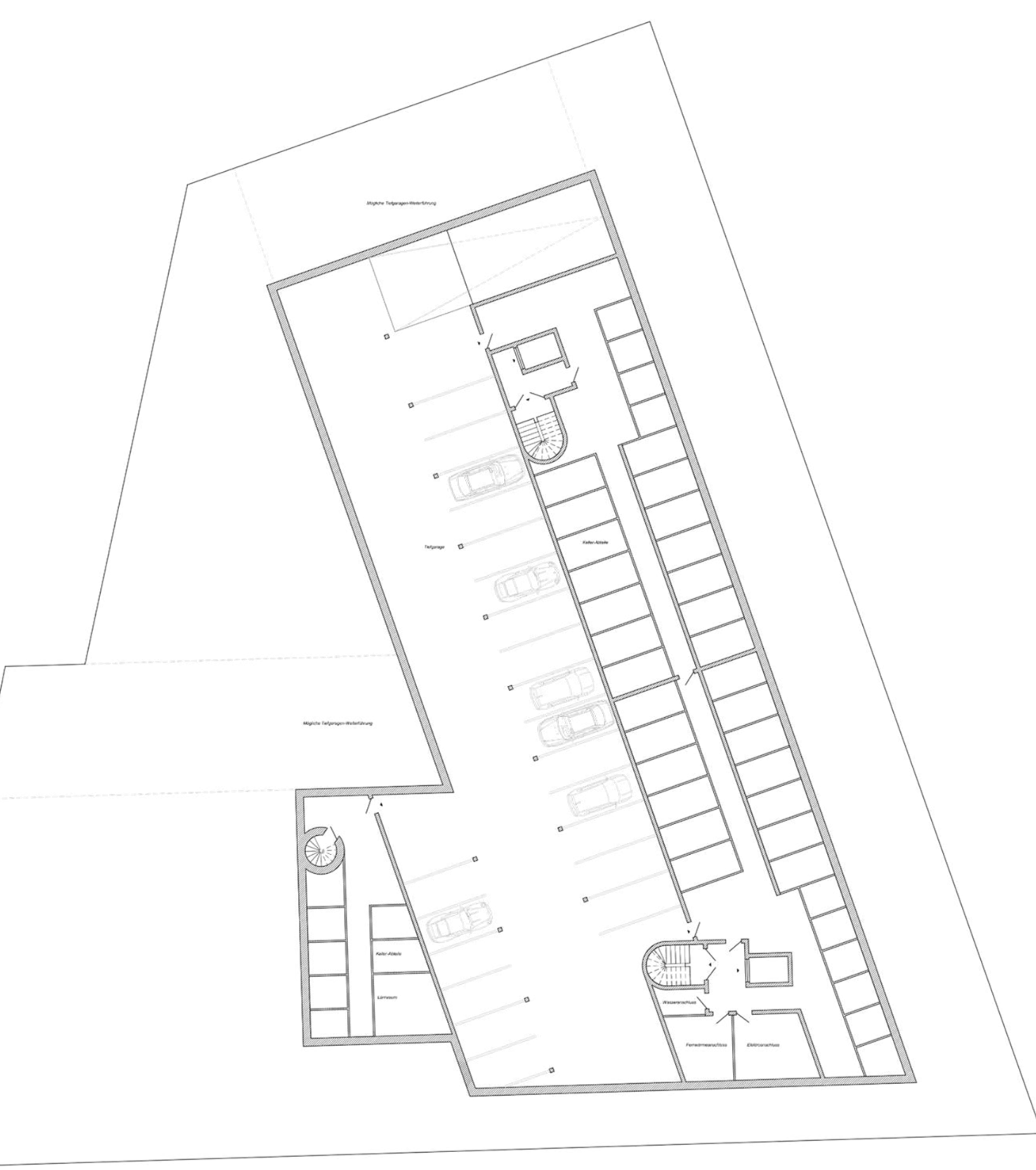
Grundriss Untergeschoss M 1:200
