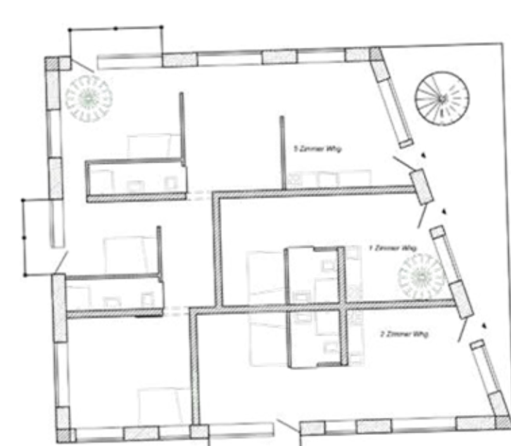
Grundriss 2. Obergeschoss M 1:200
