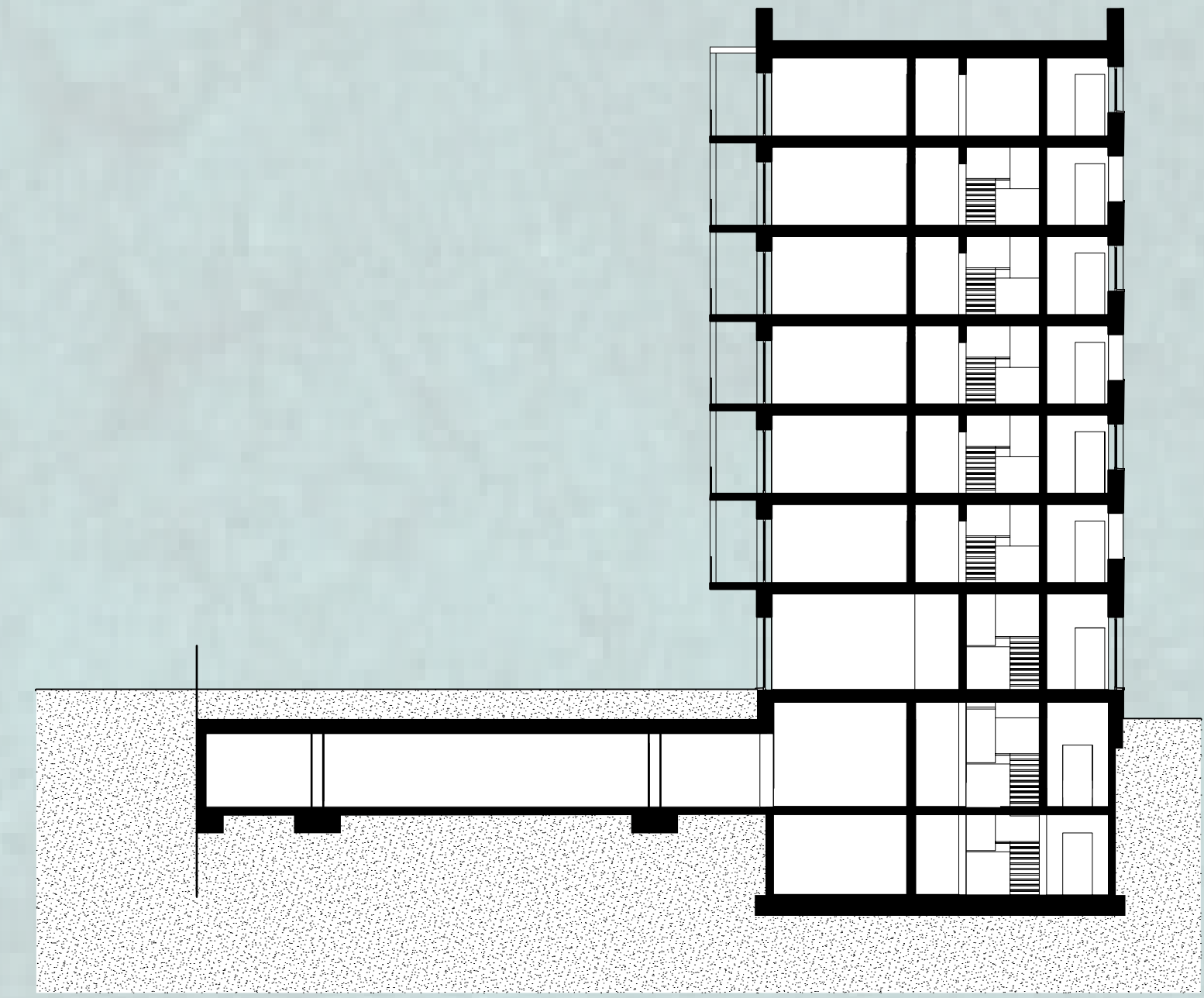
Schnitt 1:200
