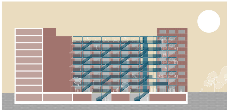
Ansicht Konsekutivtreppe
