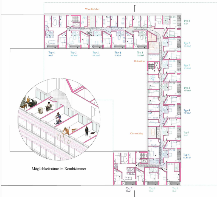
Korridorlage im 2./5. OG // MI:200
